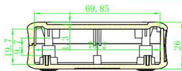
SEC A-A
