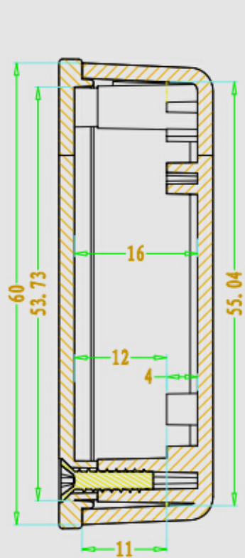
SEC A-A
