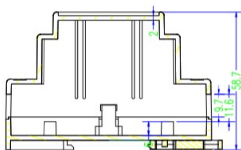
剖面 2-2
